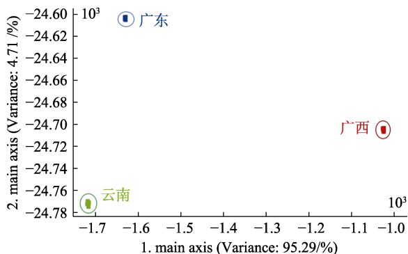
图 8 LDA 分析图
