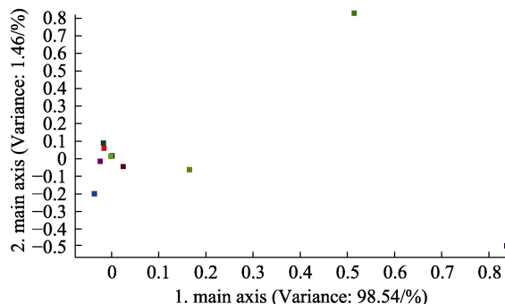
图 10 Loading 分析图
